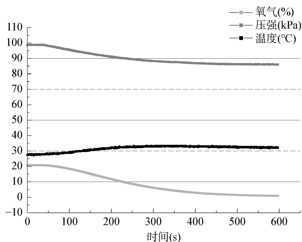
图8 “暖宝宝”内芯氧化引发的氧气含量、温度和压强变化
