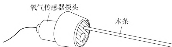
图 3 氧气传感器探头及木条安装细节图
