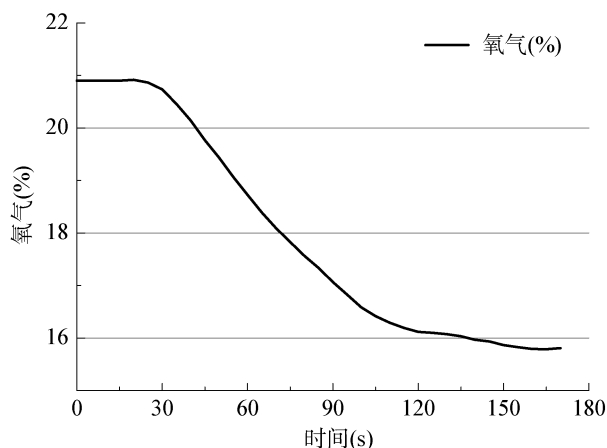
图6 蜡烛燃烧过程中的氧气含量变化
