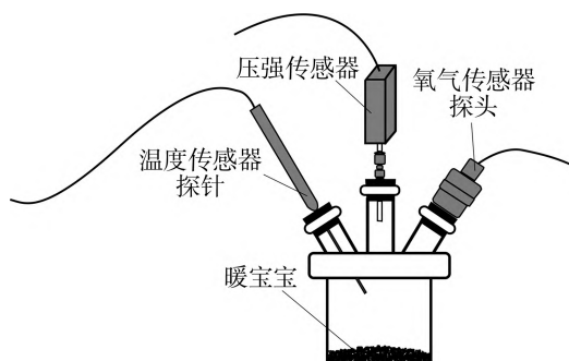
图7 将三种传感器接入三口分体烧瓶
