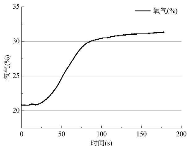
图 10 加入过氧化氢后,锥形瓶内氧气含量上升
