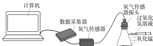
图9 测量过氧化氢分解过程中氧气含量的实验装置
