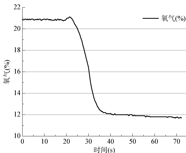
图 4 木条燃烧后引起集气瓶内氧气含量下降
