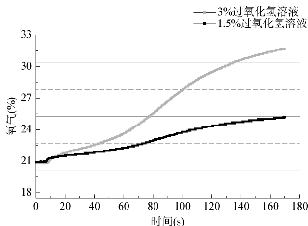
图 11 溶液浓度对过氧化氢分解产生氧气的影响
