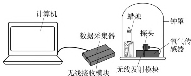
图 5 使用氧气传感器测量蜡烛燃烧导致的氧气含量变化
